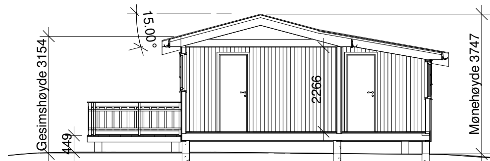
SNITT 1 : 100
