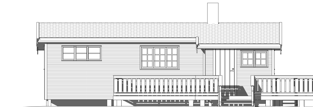
Fasade Sør
